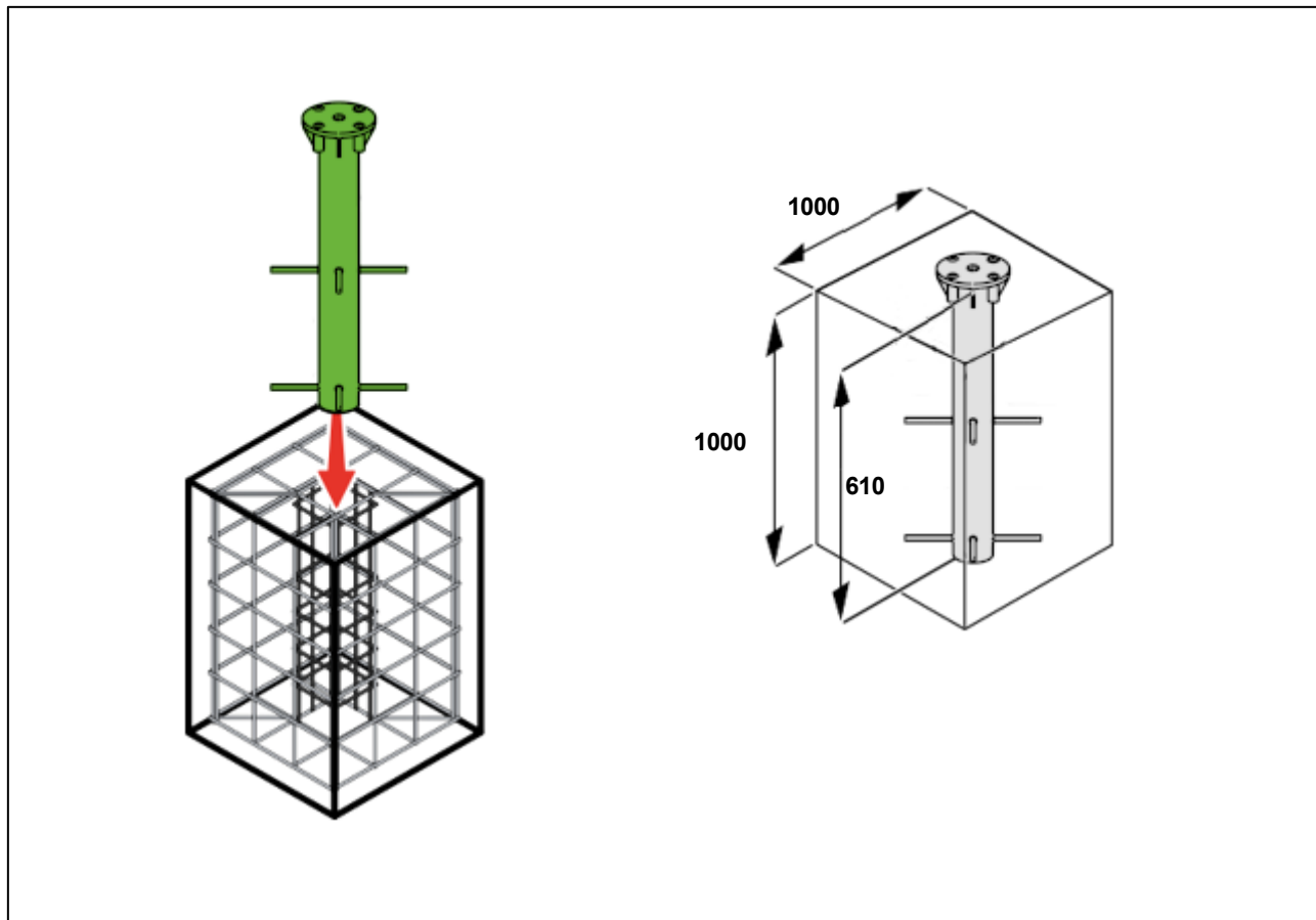
Fig. 6 : Procédure pour sceller la douille de sol dans le béton
