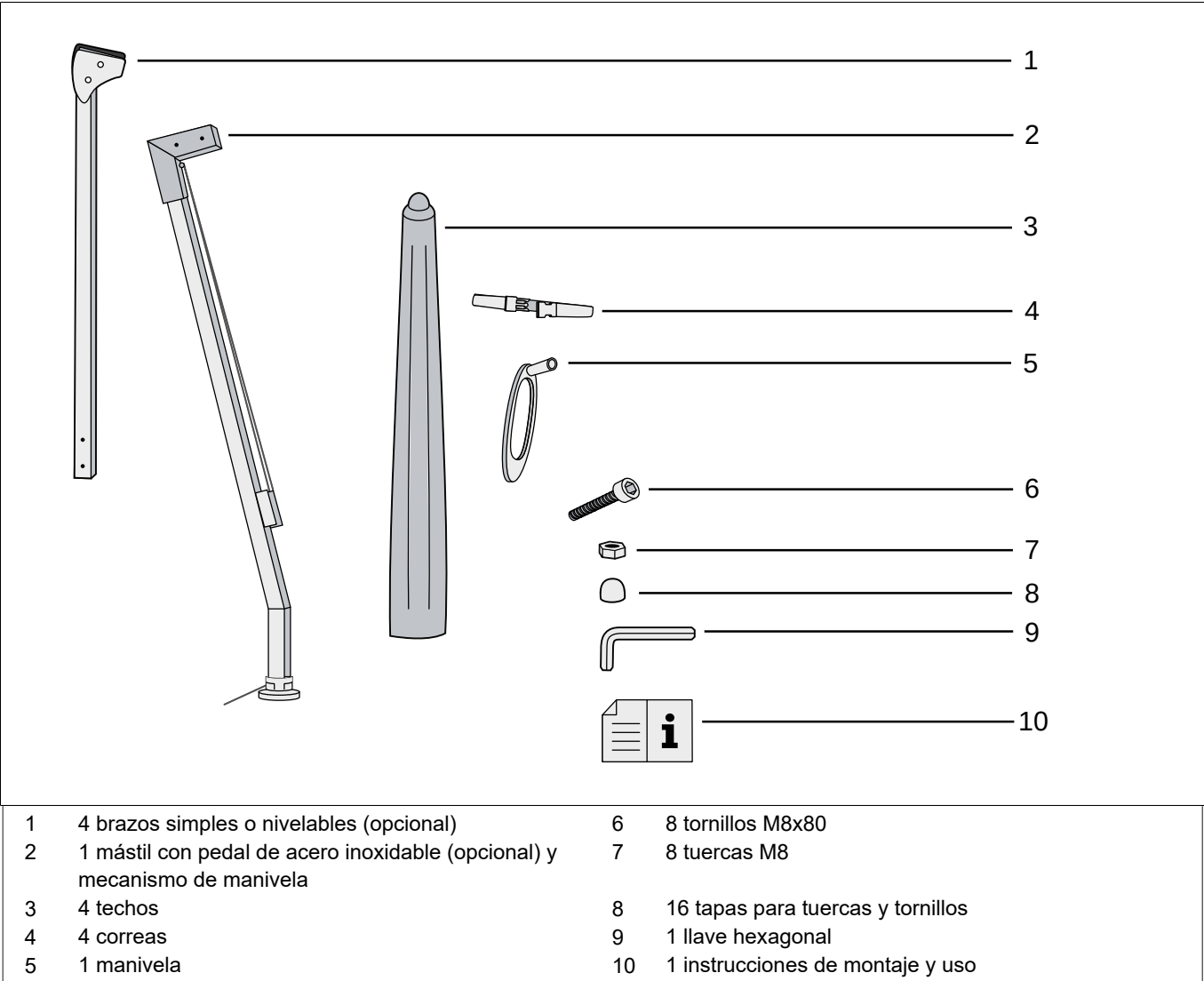
Fig. 17: Volumen de suministro Amalfi Quadro
