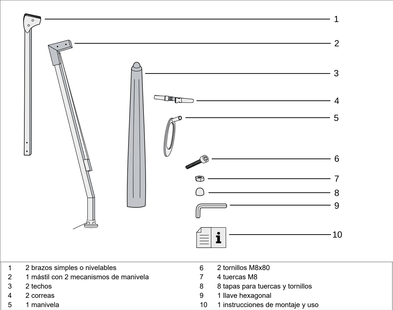
Fig. 16: Volumen de suministro Amalfi Duo
