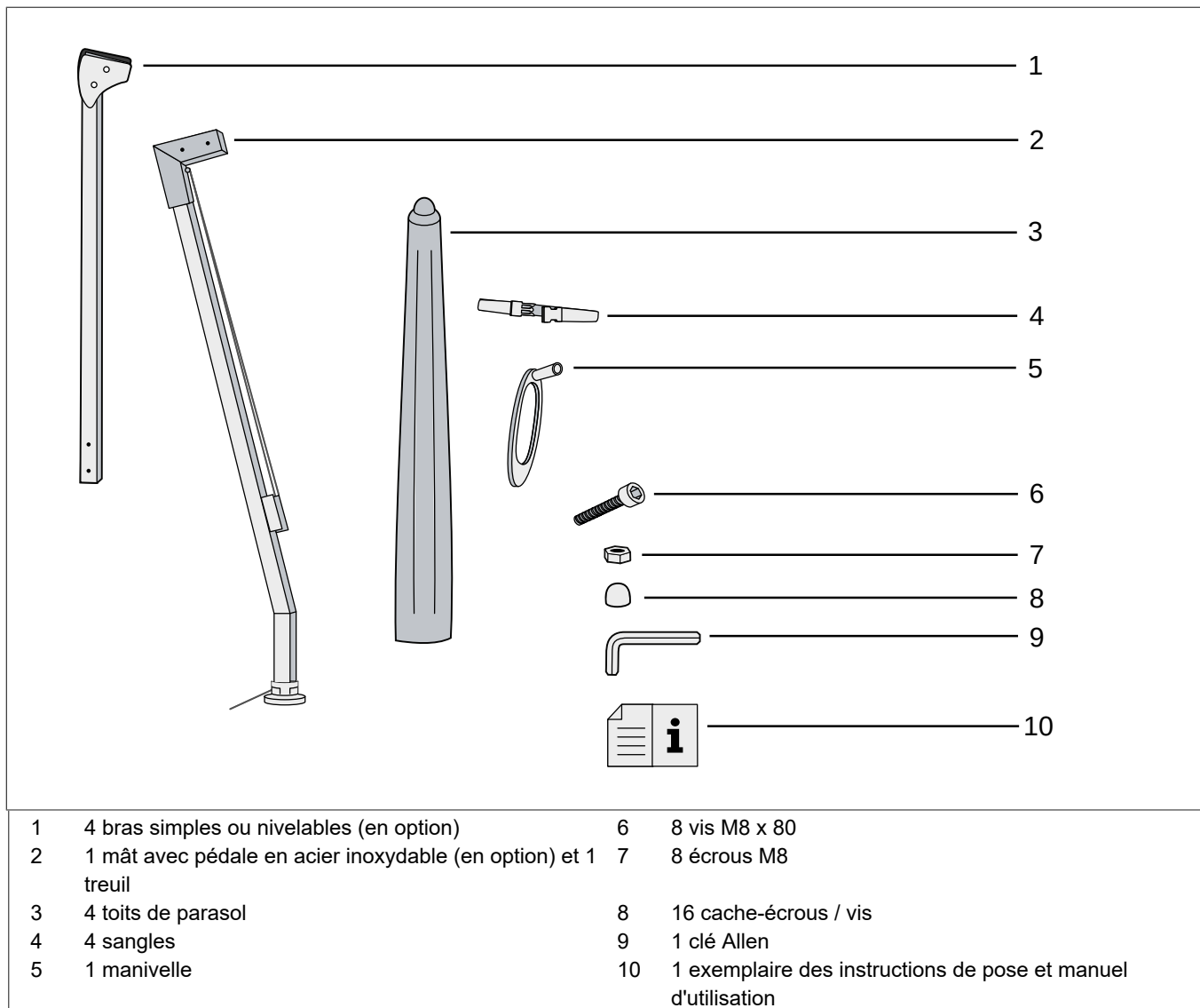
Fig. 12: Volume de livraison Amalfi Quadro
