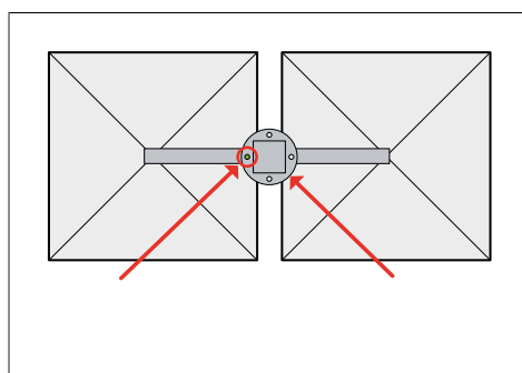
Fig. 13: Alignement des trous filetés d'un DUO 1
