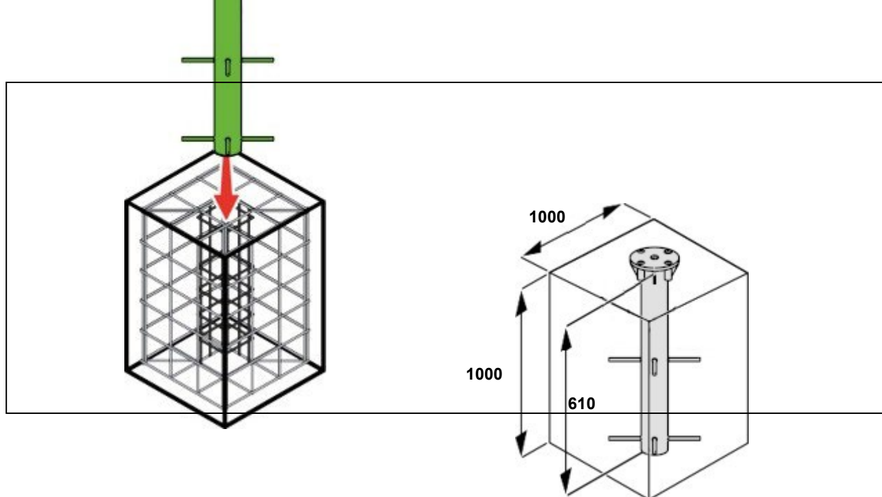
Fig. 6 : Procédure d'encastrement de la douille dans le béton
