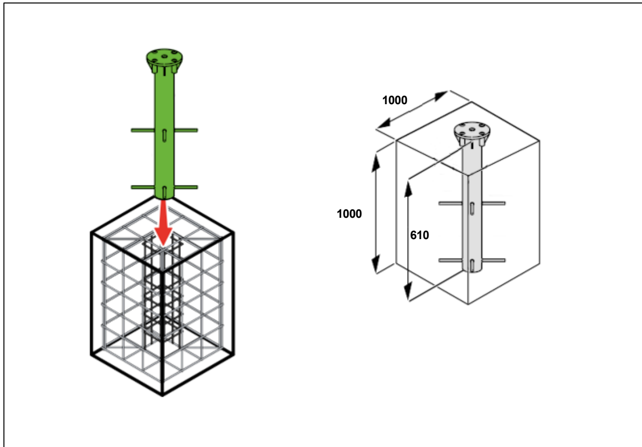
Abb. 6: Vorgehen Bodenhülse einbetonieren
