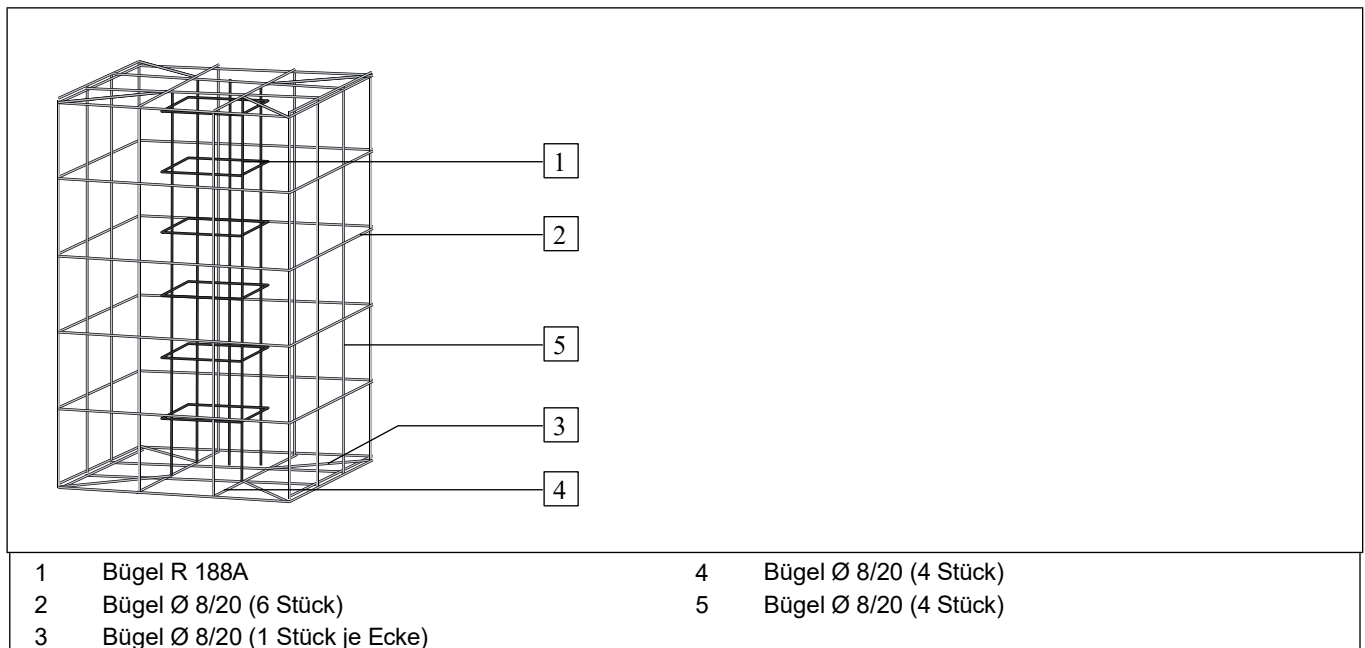
Abb. 2: Bewehrung binden
